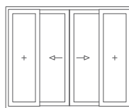
Vierteiliges Element mit zwei Schiebeflügeln und zwei Festverglasungen außen.
